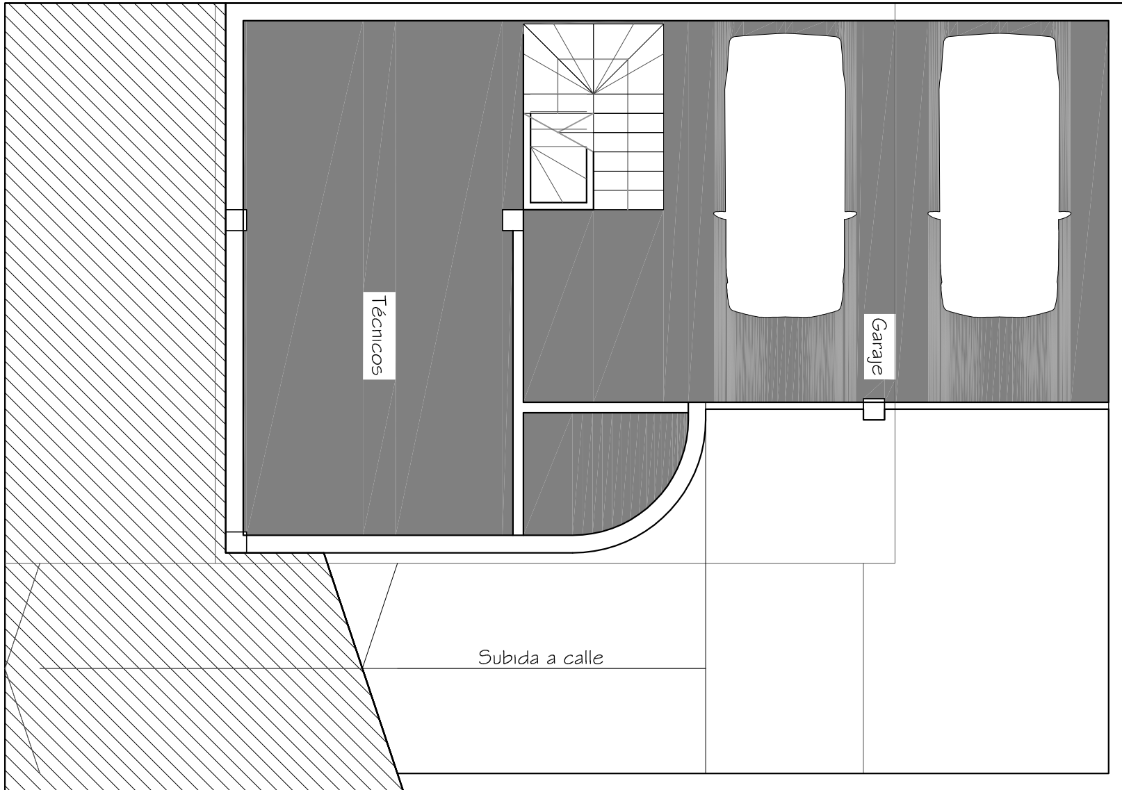
MODELO 3B / PAREADO_UNIFAMILIAR Garaje en Sótano E 1/75
