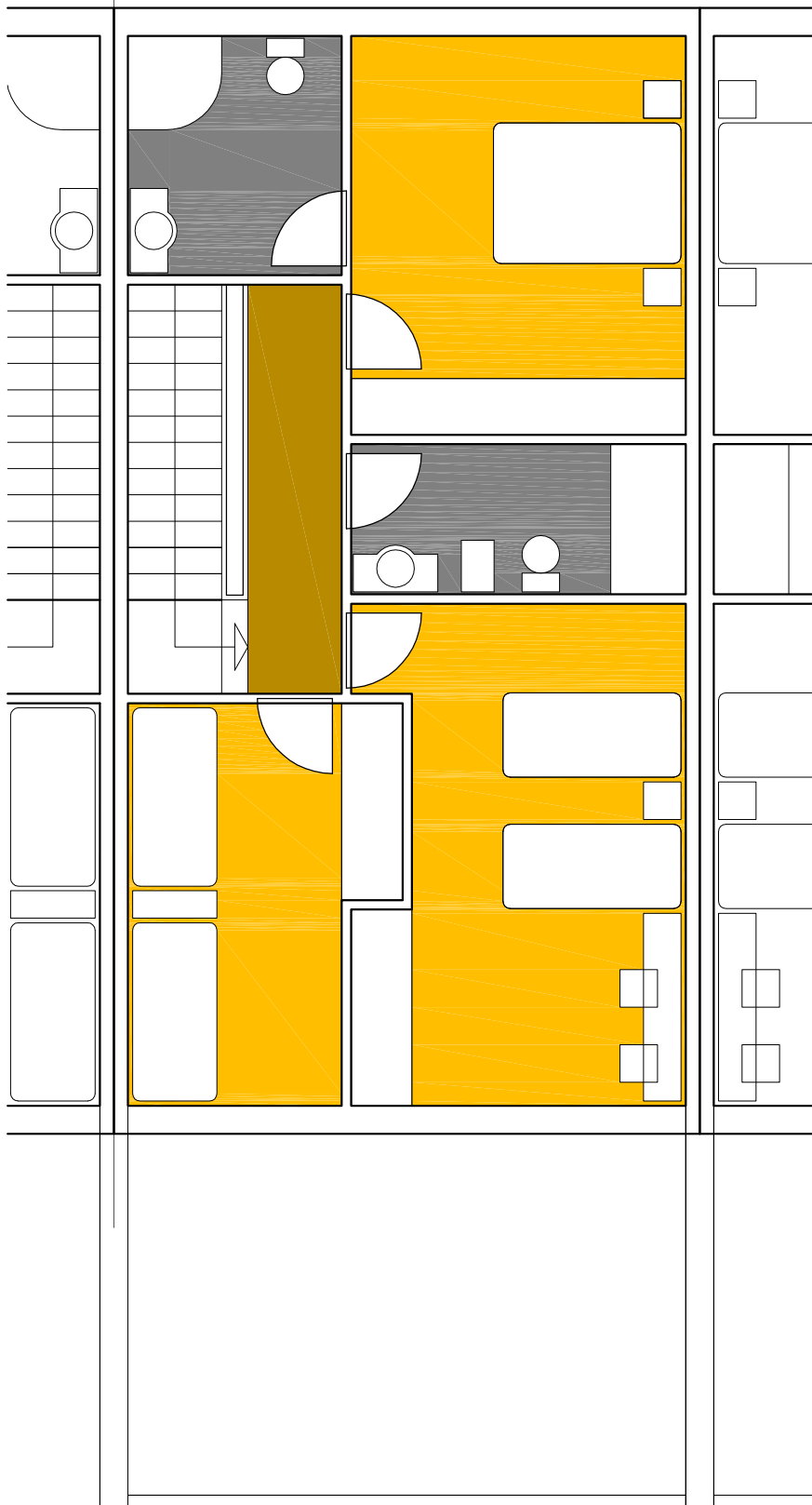
MODELO 2B ADOSADO / UNFAMILIAR PLANTA SEGUNDA E 1 / 75
