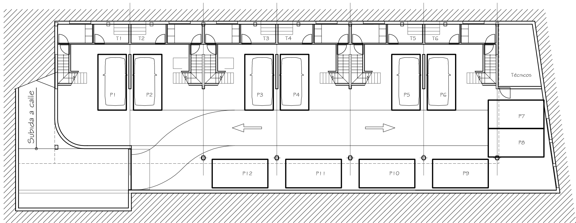
MODELO 2A / ADOSADOS SÓTANO / Garaje mancomunado E 1/200
